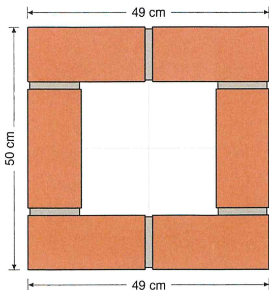
Pianta 1ª Fila (Ingombro 49x50 cm)
