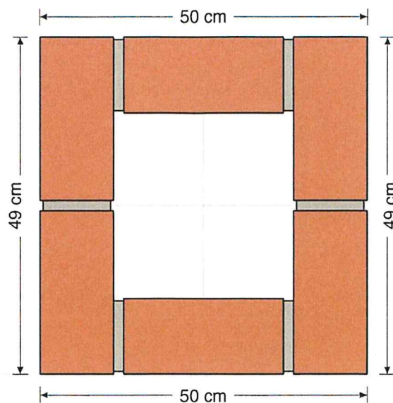
Pianta 2ª Fila (Ingombro 50x49 cm)
